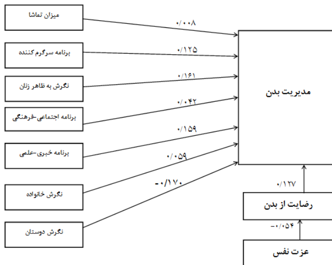
نمودار شماره‌ی دو- تحلیل مسیر میزان مدیریت بدن
